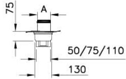
Altın çıkışlı kesit
