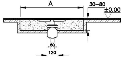
Altın Çıkışlı Sifon Kesit
